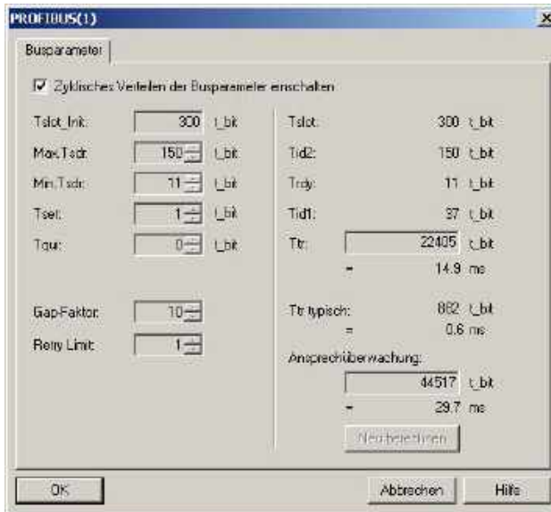
Abbildung 11: Zyklisches Verteilen der Busparameter
