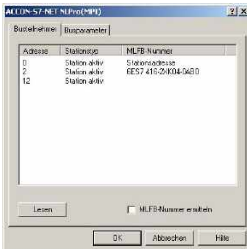
Abbildung 14: Diagnosefunktion
