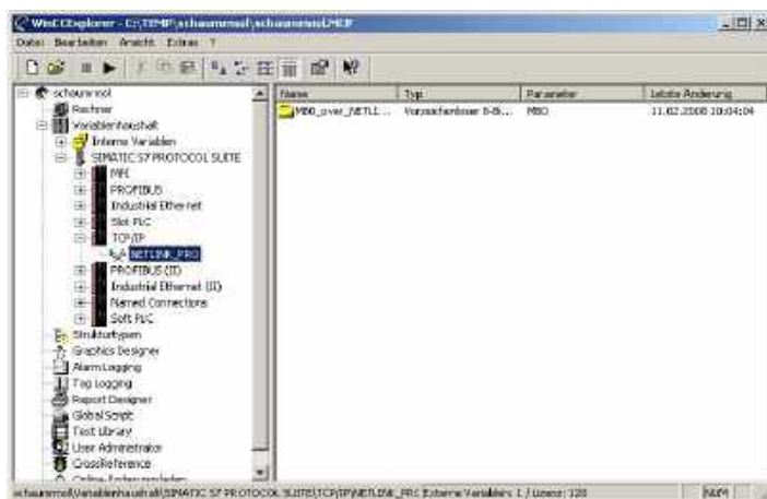
Abbildung 21: Verbindung »NETLINK_PRO«
