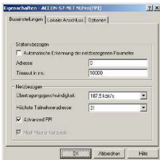
Abbildung 12: Buseinstellungen PPI
