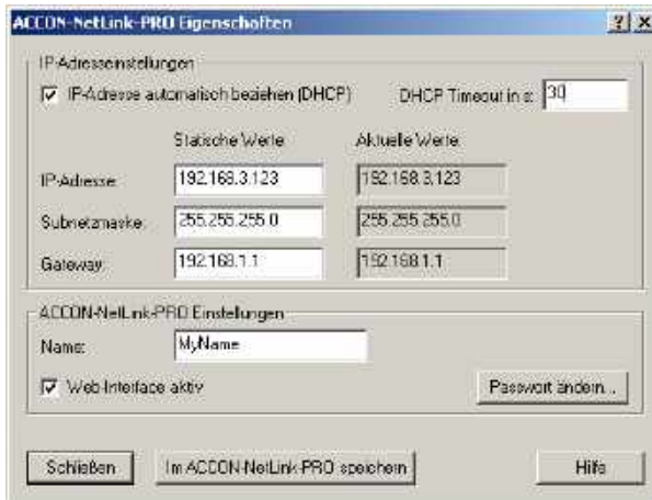
Abbildung 7: Einstellungen im ACCON-NetLink-PRO compact
