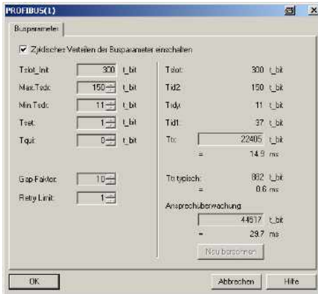
Abbildung 7: Zyklisches Verteilen der Busparameter
