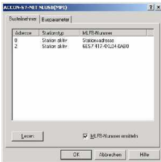
Abbildung 10: Diagnosefunktion
