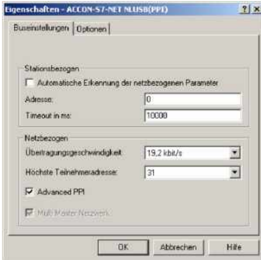
Abbildung 8: Buseinstellungen PPI
