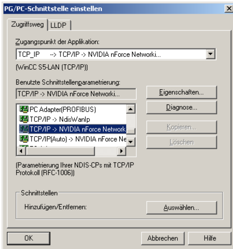
Abbildung 23: PG/PC-Schnittstelle einstellen
