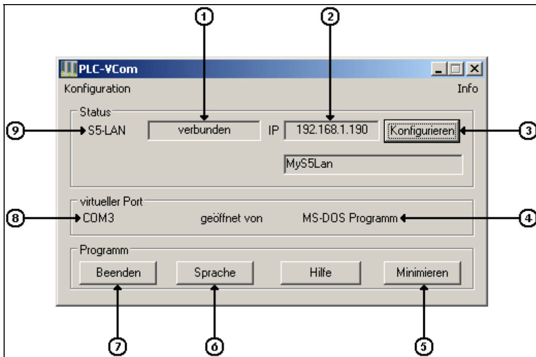
Abbildung 7: PLC-VCom Dialog
