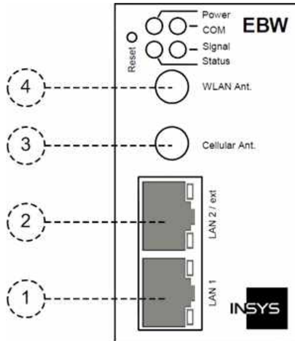
Abbildung 2: Anschlüsse auf der Gerätevorderseite
